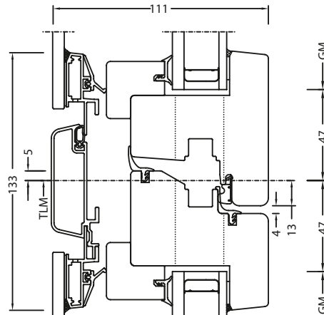
Schnitt waagrecht
