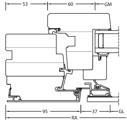
Schnitt Stulp
