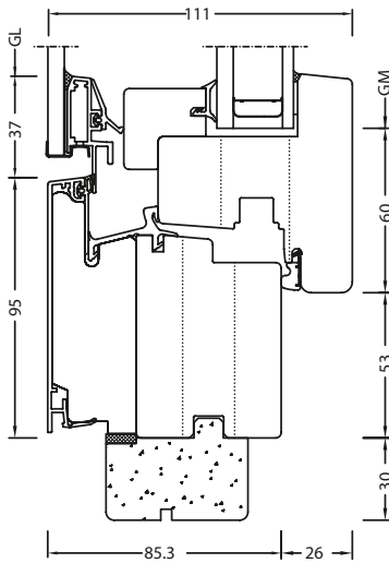
Schnitt senkrecht
