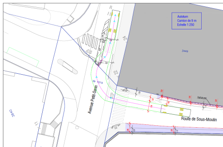
Aménagement détail
