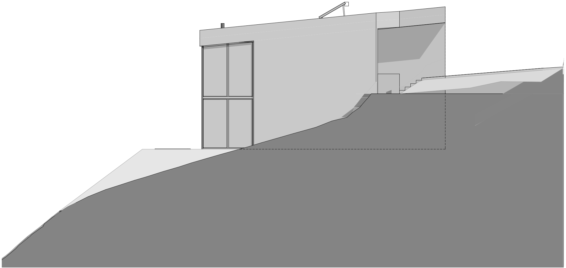
Façade Est_1:100
