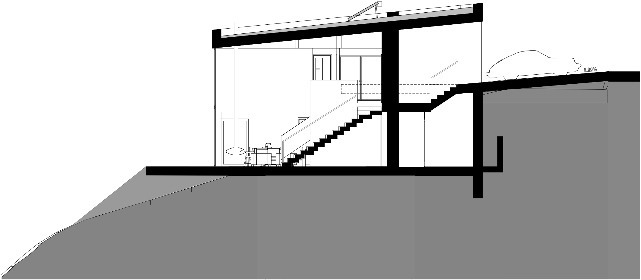
Coupe A-A'_1:100
