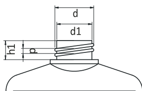
ZE-Gewinde / K-Gewinde
