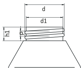
CT-Gewinde
