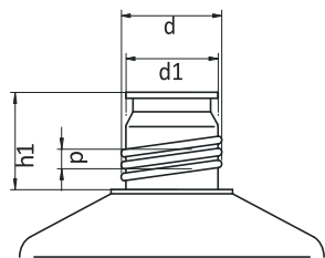
JK-Gewinde
