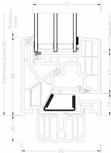
Schnitt senkrecht
