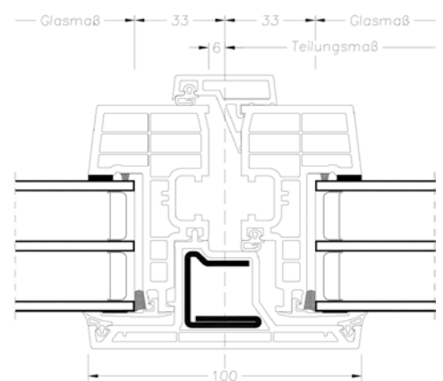
Schnitt Stulp
