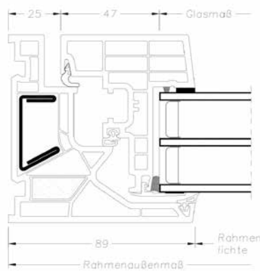
Schnitt waagrecht
